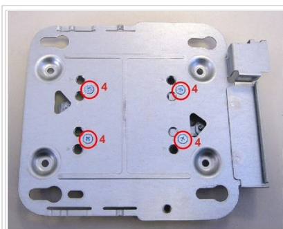
Fig. 7 - Fijación de la platina
