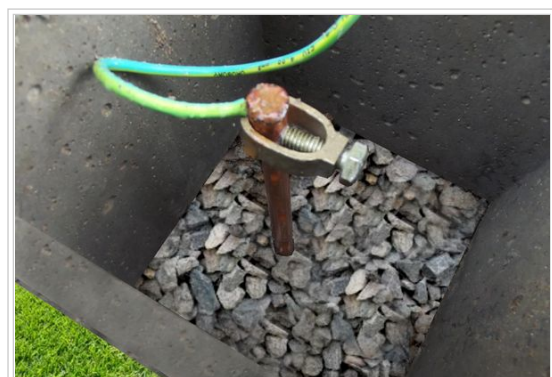
Fig. 2 : Cámara de puesta a tierra
