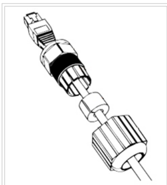
Fig. 3 - Enhebrado de prensacable (fuente: manual Ruckus)
