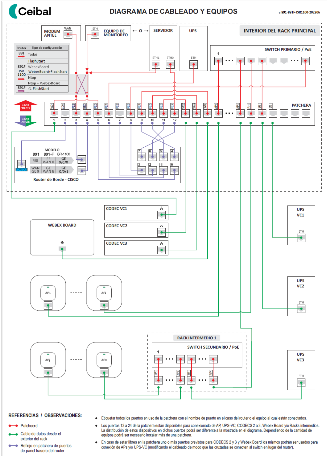
Fig. 1 - Diagrama de interconexión de equipos con router Cisco 891 / 891F / ISR-1100.
