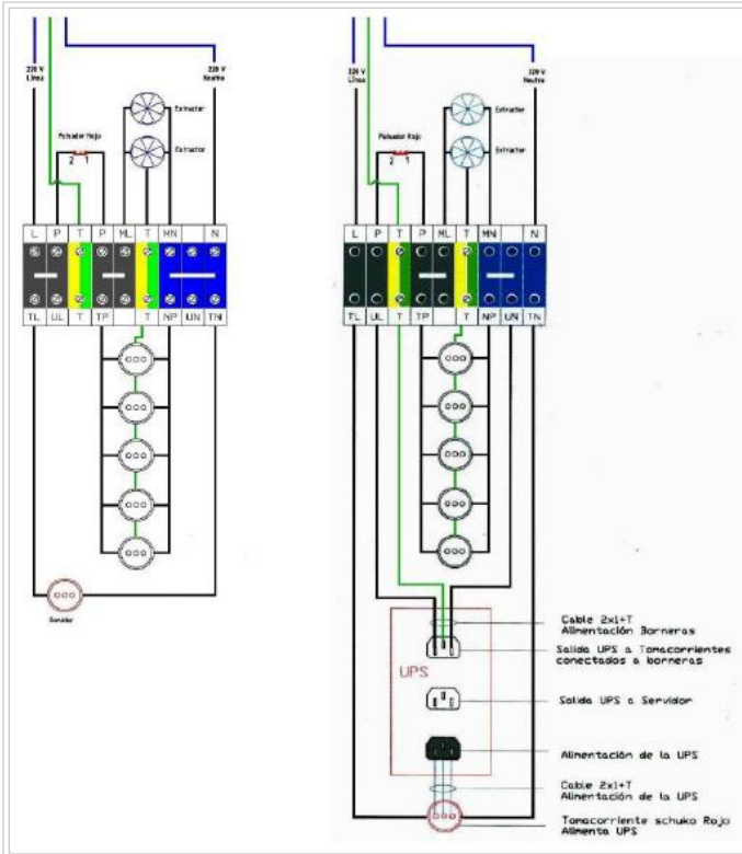
Fig. 5 : Diagrama eléctrico de bandeja con bornera
