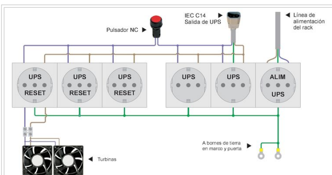
Fig. 7 : Diagrama eléctrico de bandeja sin bornera
