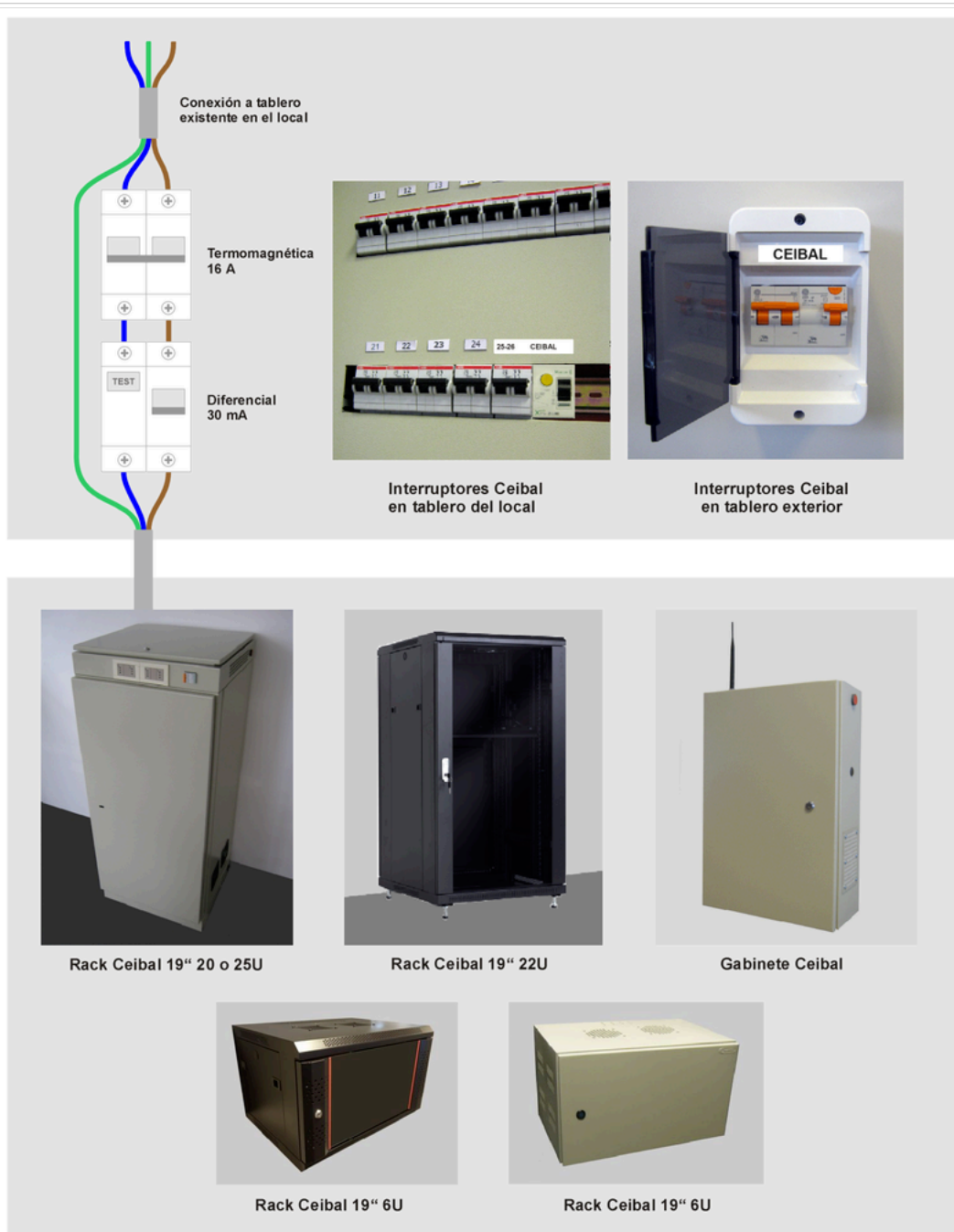
Fig. 1 - Esquema general de la instalación eléctrica
