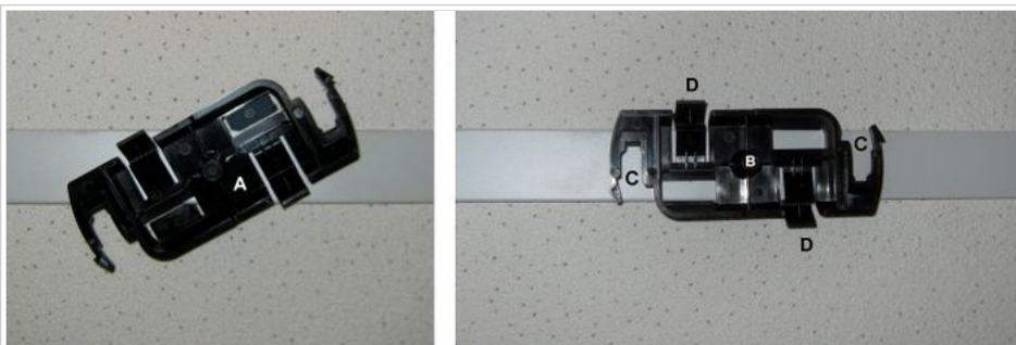
Fig. 4 - Soporte Aruba para cielorraso tipo Armstrong
