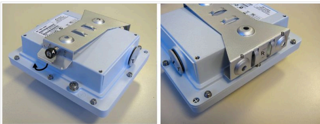
Fig. 2 - Soporte Ruckus
