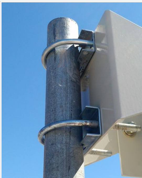
Fig. 3 - Fijación del soporte al caño
