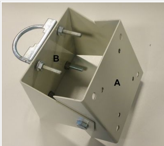
Fig. 2 - Soporte
