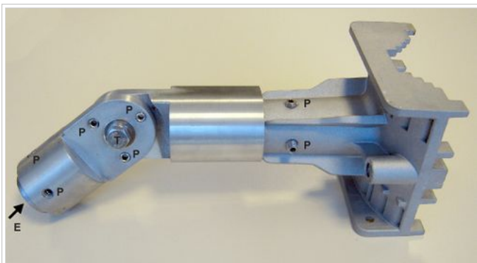
Fig. 6 - Soporte Wavion direccional
